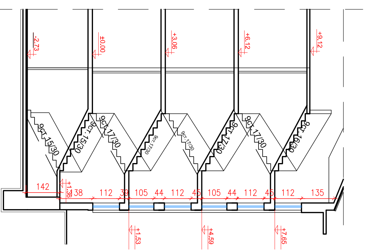
ВЕРТ.РАЗРЕЗ "Б-Б" М1:100
