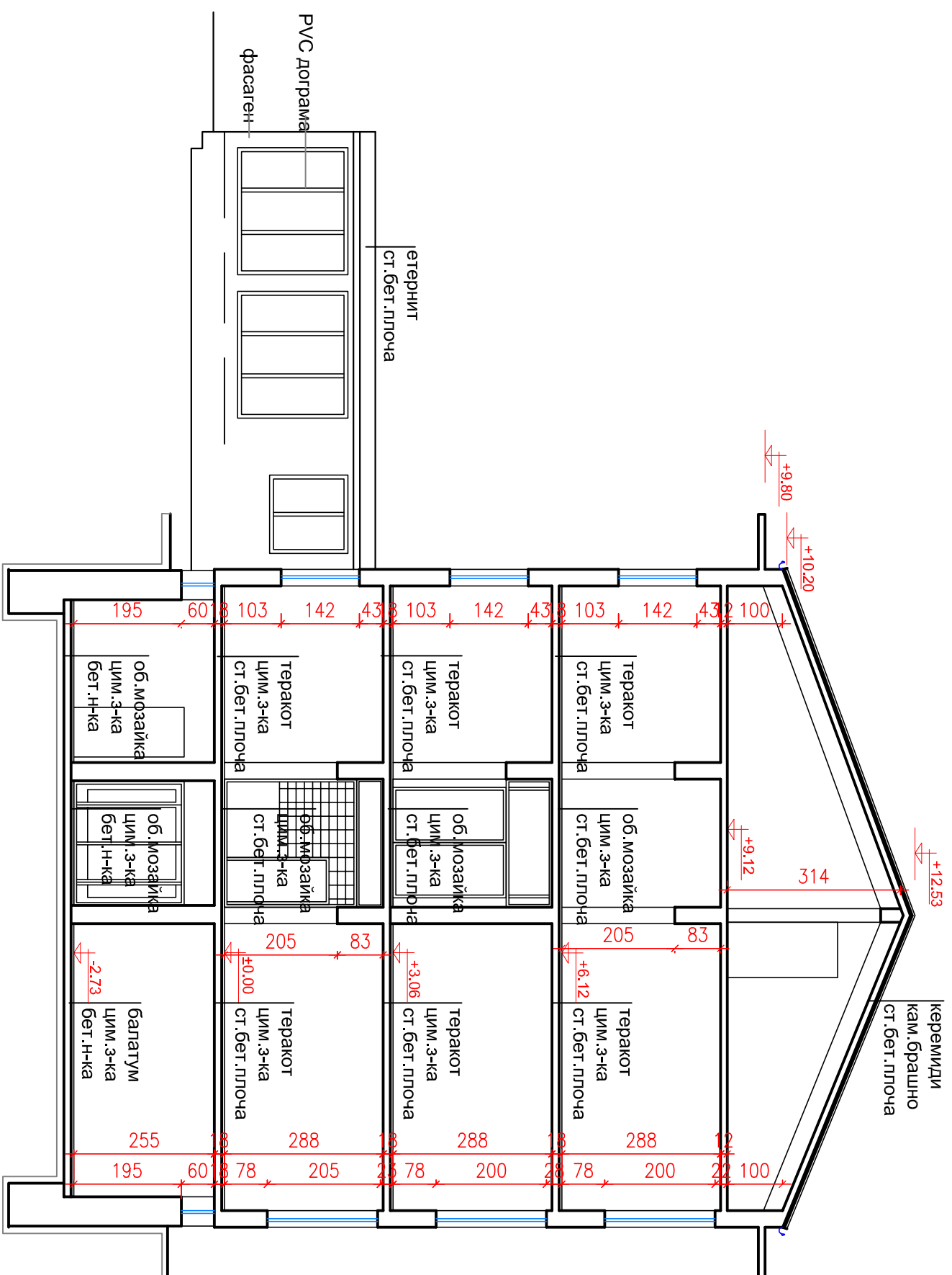
ВЕРТ.РАЗРЕЗ "А-А" М1:100
